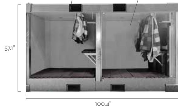
SPACE-SAVING MODULE
