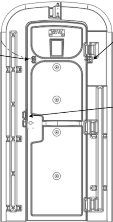
PN 19779 BRACKET- TM DOOR SPRING DOOR
